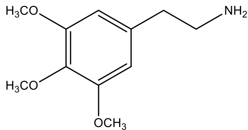
Meskalina
