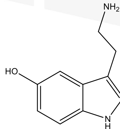
Serotonina
