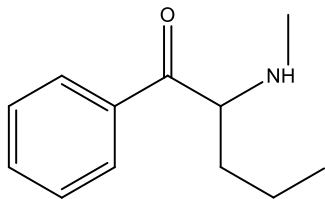
Pentedron
