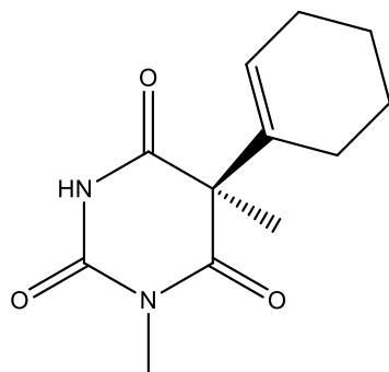
Heksobarbital
