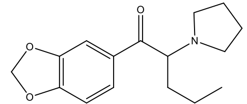
MDPV
