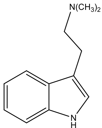
Dimetylotryptamina DMT
