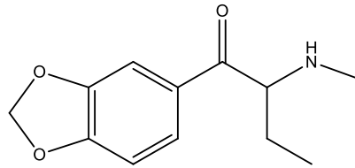
Butylon, bk-MBDB
