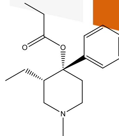
Alfameprodyna
