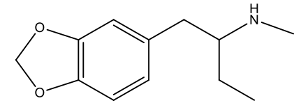
MBDB - Eden
