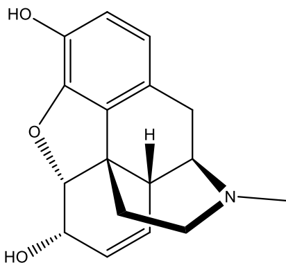
Morfina
