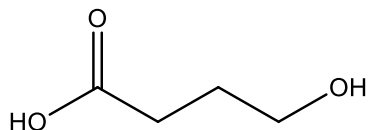
GHB
