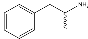
Amfetamina
